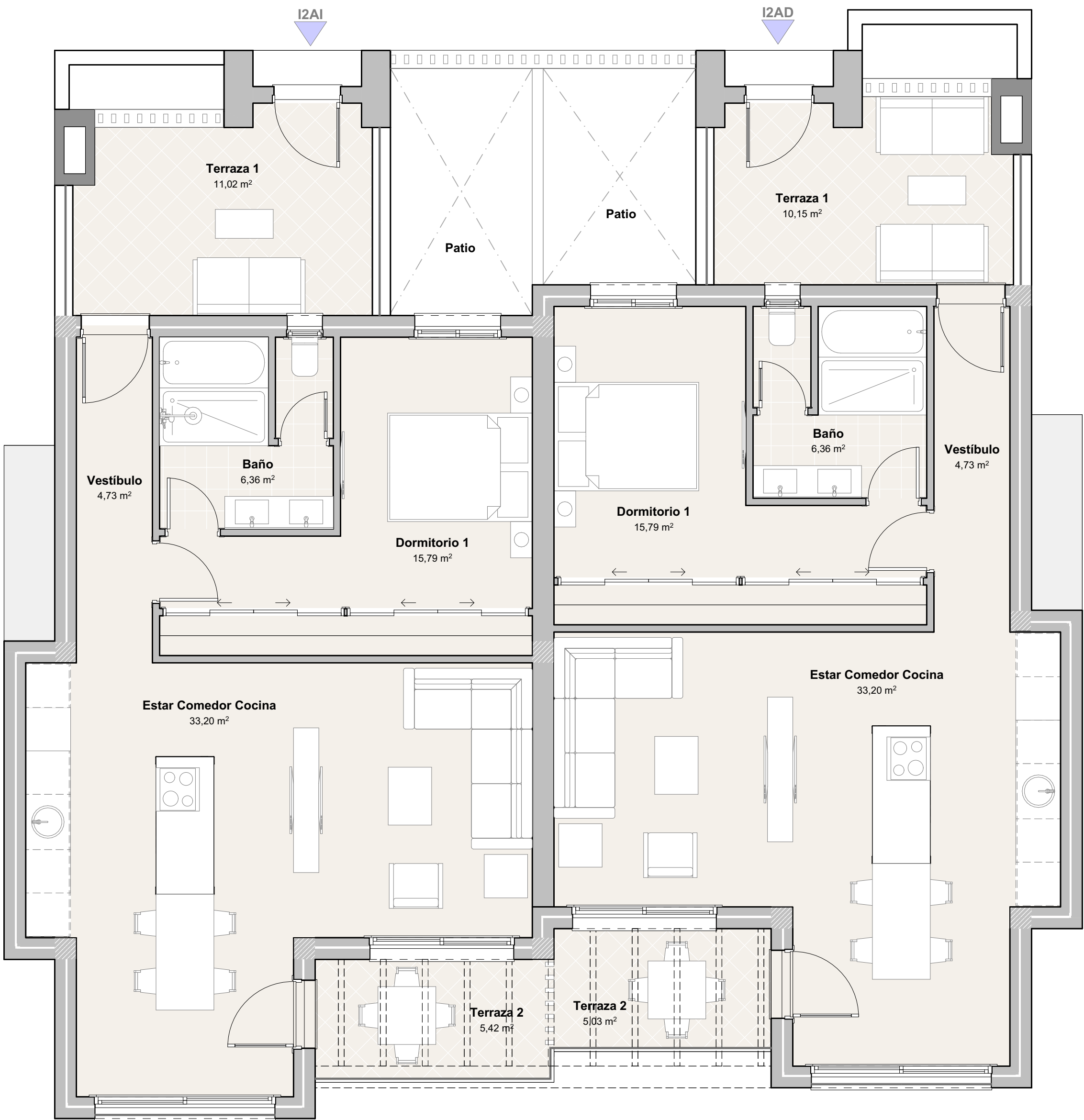
Planta Viviendas Tipo I-2 I-2. Distribución, Superficies, Mobiliario 1:50
