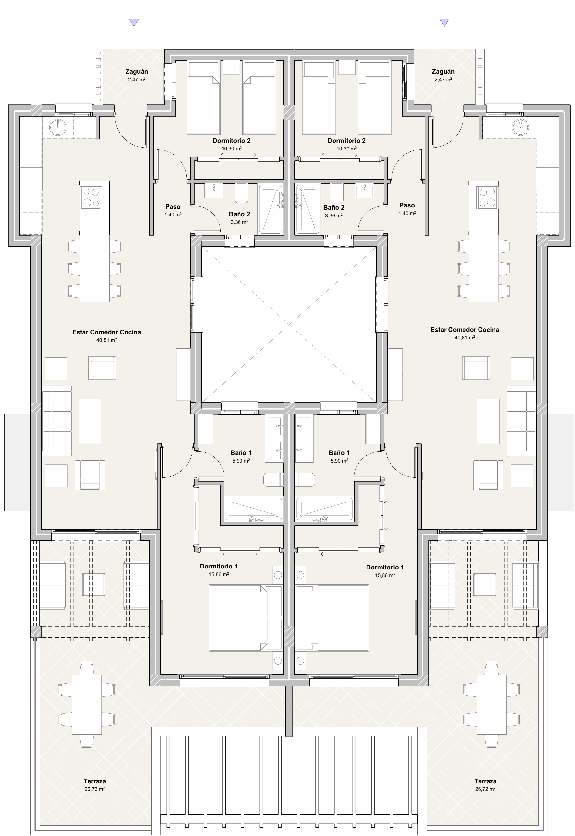
Planta Segunda Viviendas Tipo E3. Distribución, Superficies, Mobiliario. 1:50
