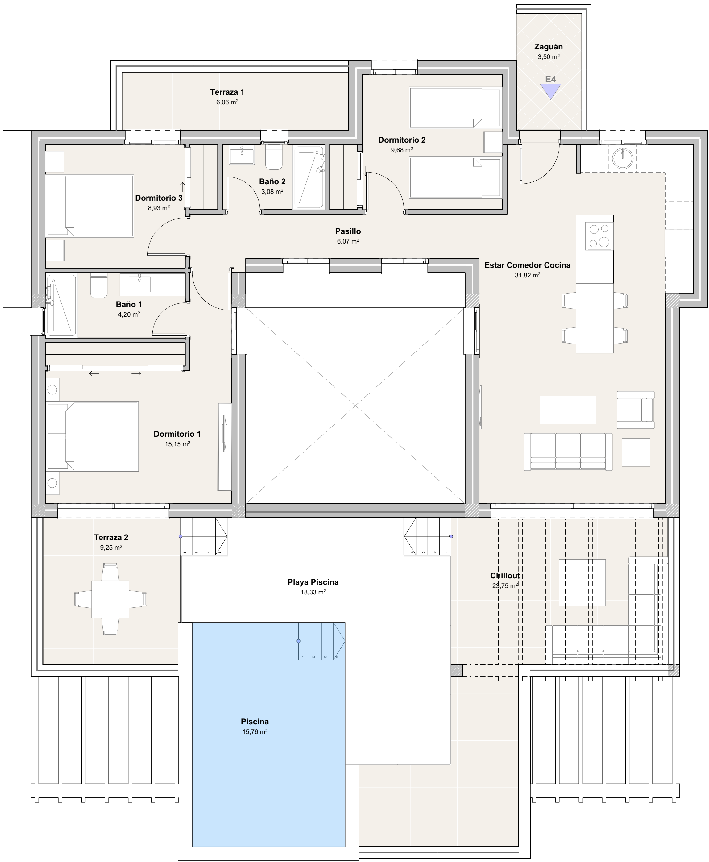
Planta Vivienda Tipo E4. Distribución, Superficies, Mobiliario. 1:50
