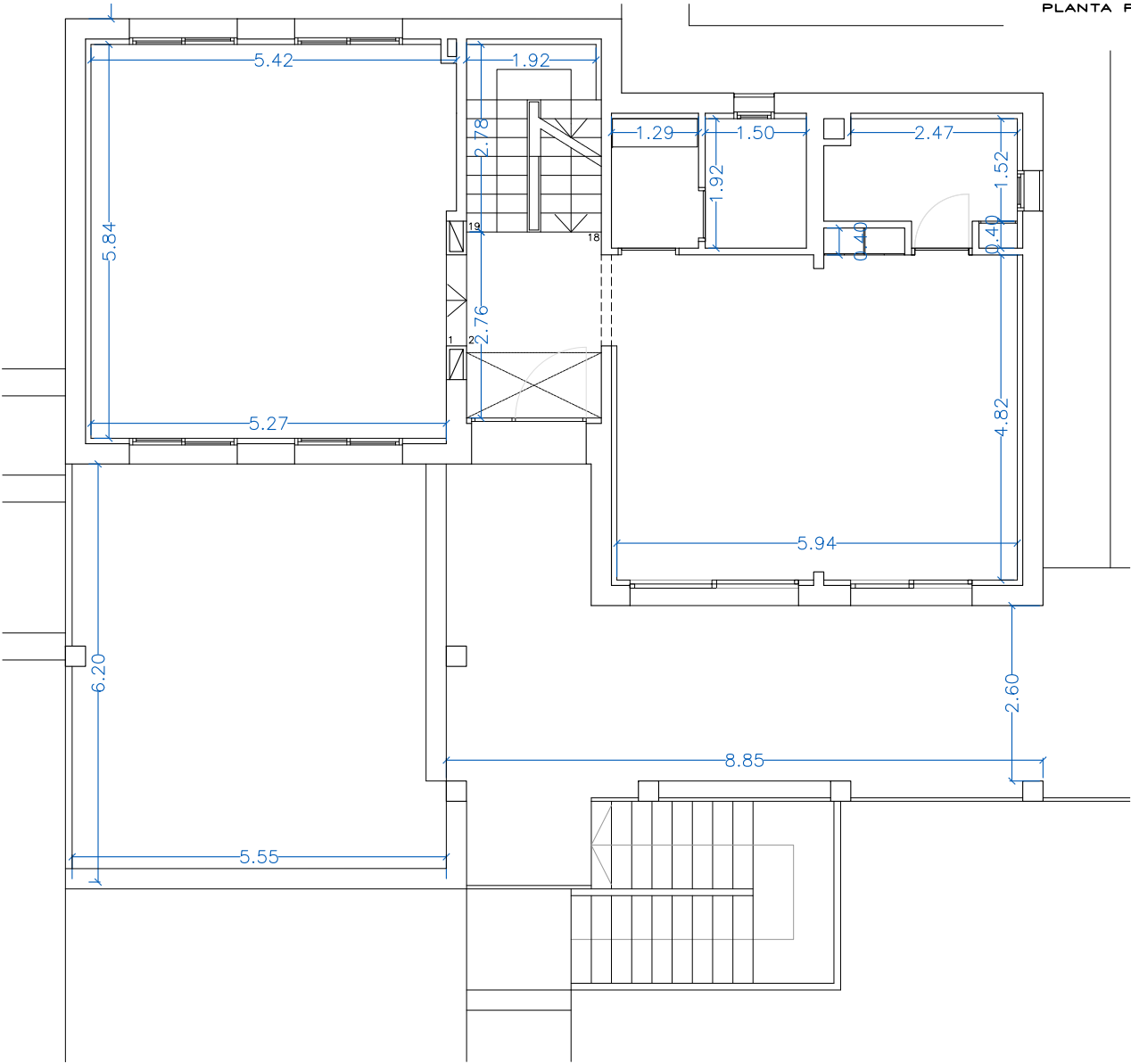
PLANTA BAJA
