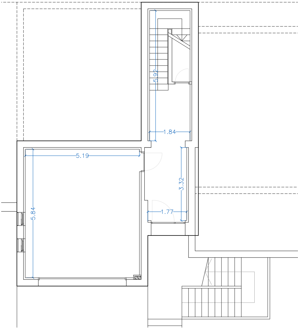
PLANTA SÓTANO
